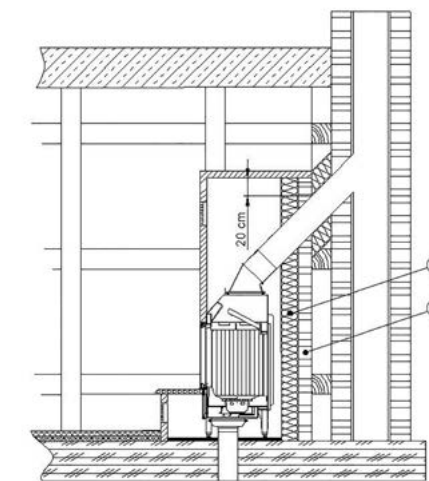
8 Dämmung der Heizkammer gemäß den Wärmedämmstoffdicken der technischen Daten 23 Vormauerung, 10 cm stark*
